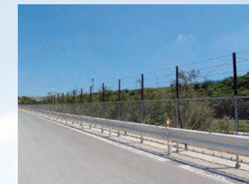
新東名 浜北 立入防止柵(嵩上げ)工事
